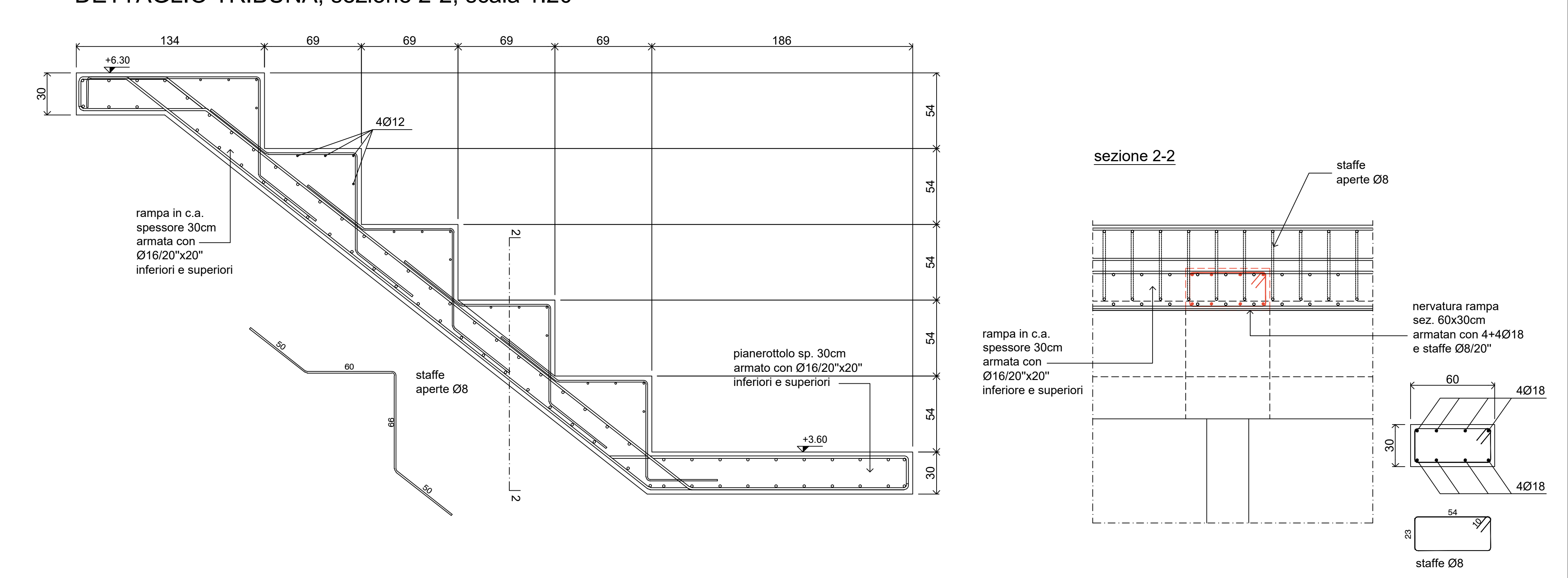
DETTAGLIO TRIBUNA sezione 2-2 scala 1:20
