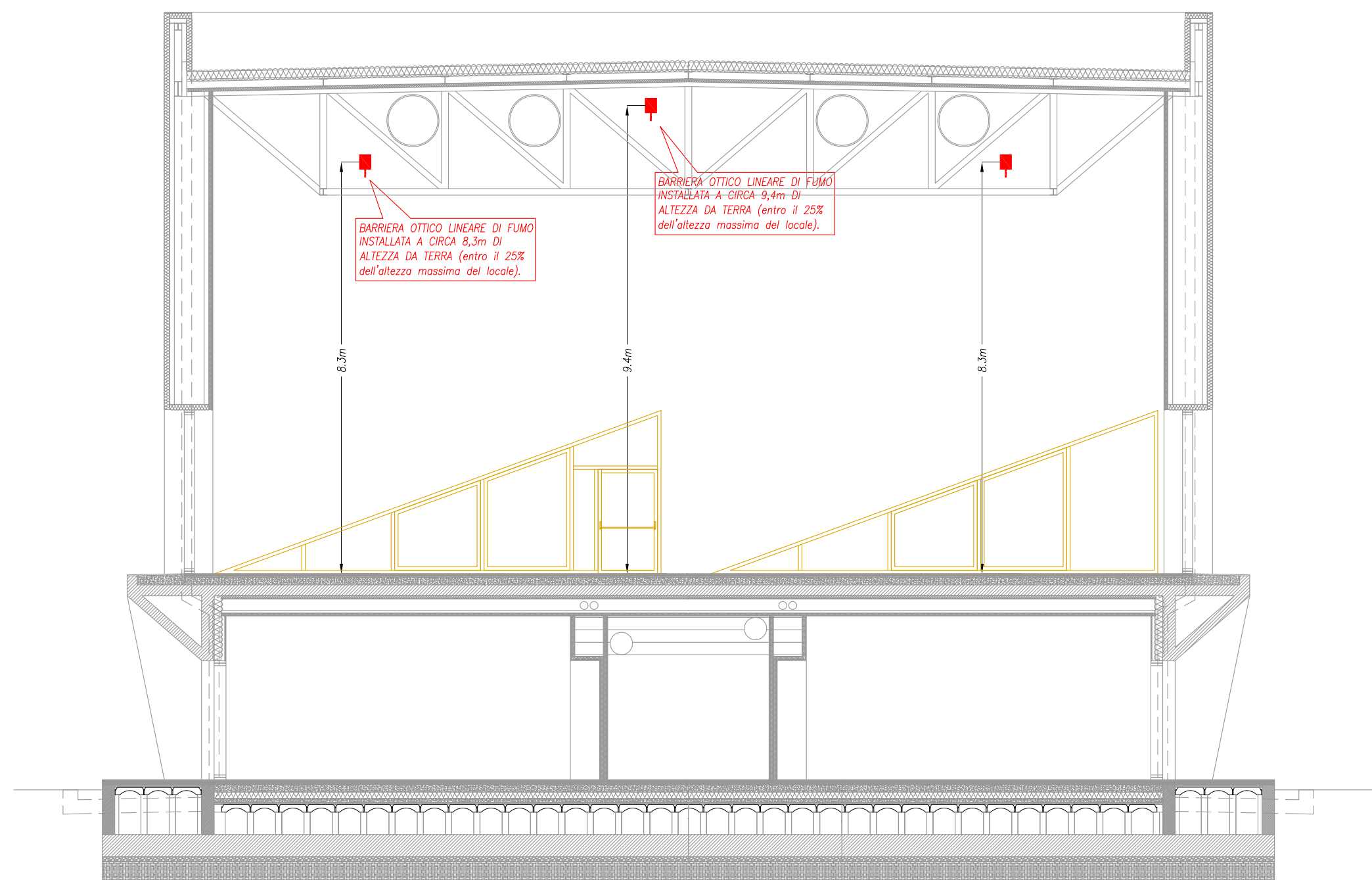
SEZIONE Scala 1:100
