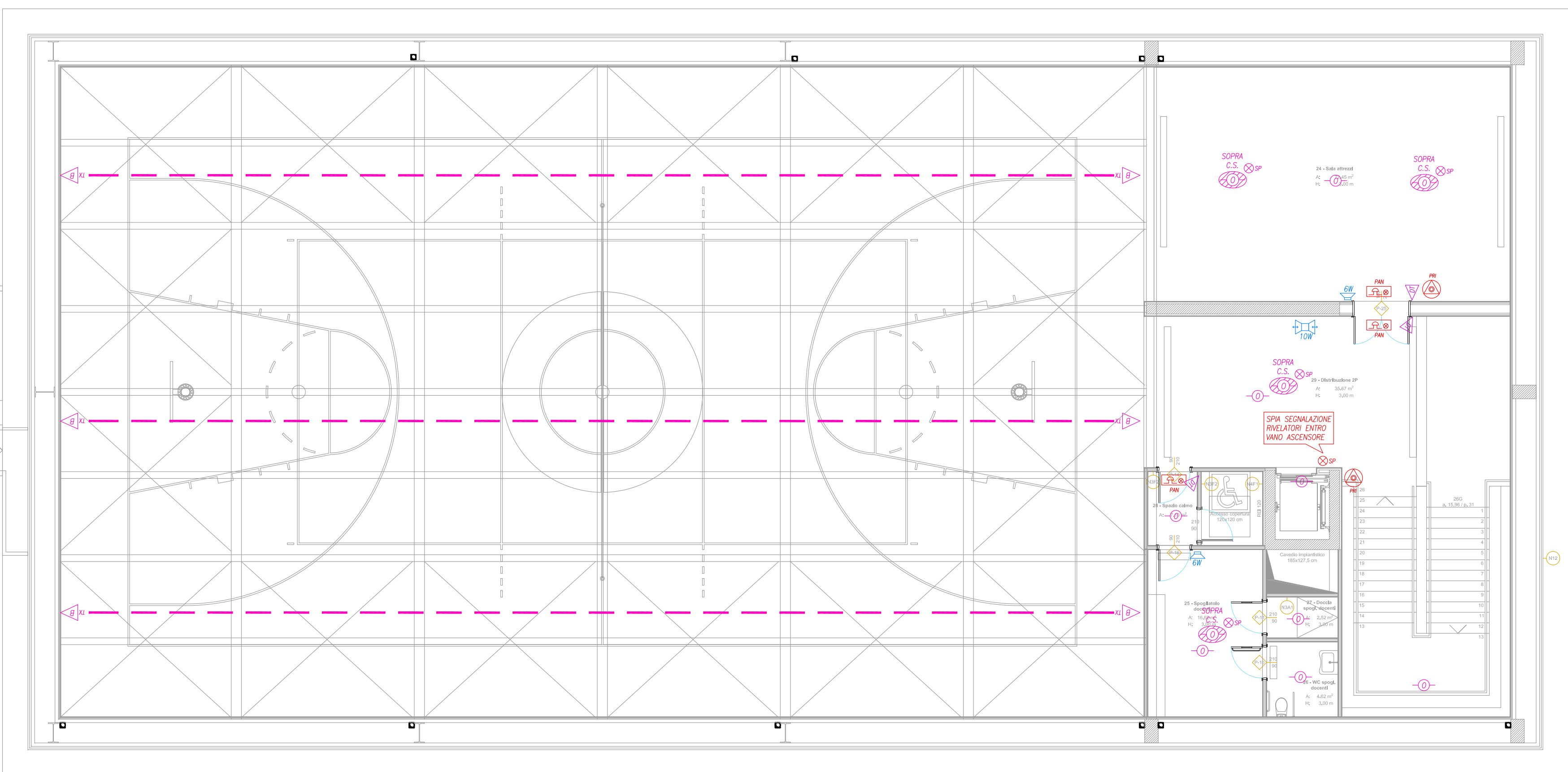
PIANO SECONDO Scala 1:100
