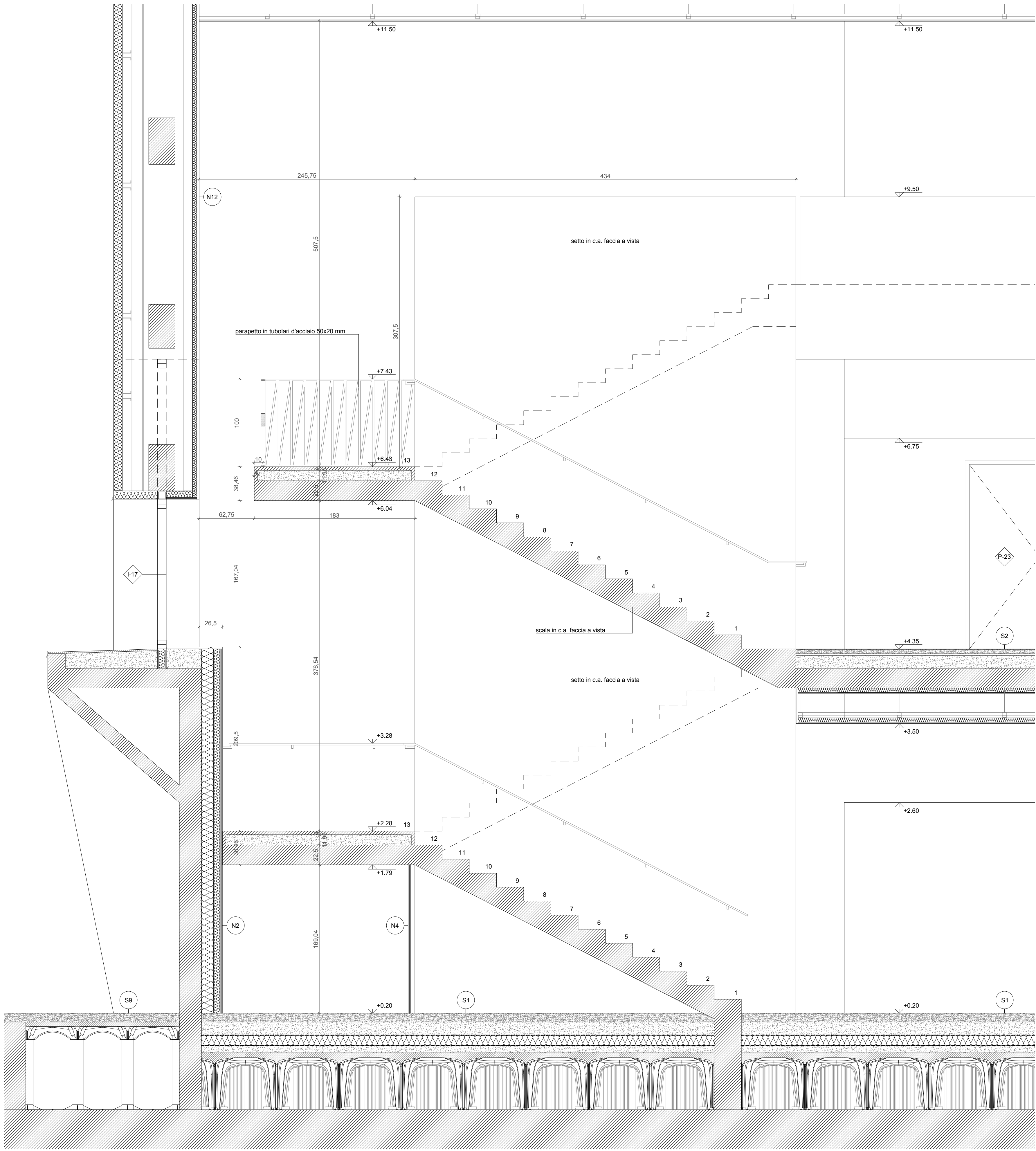
Sezione AA
