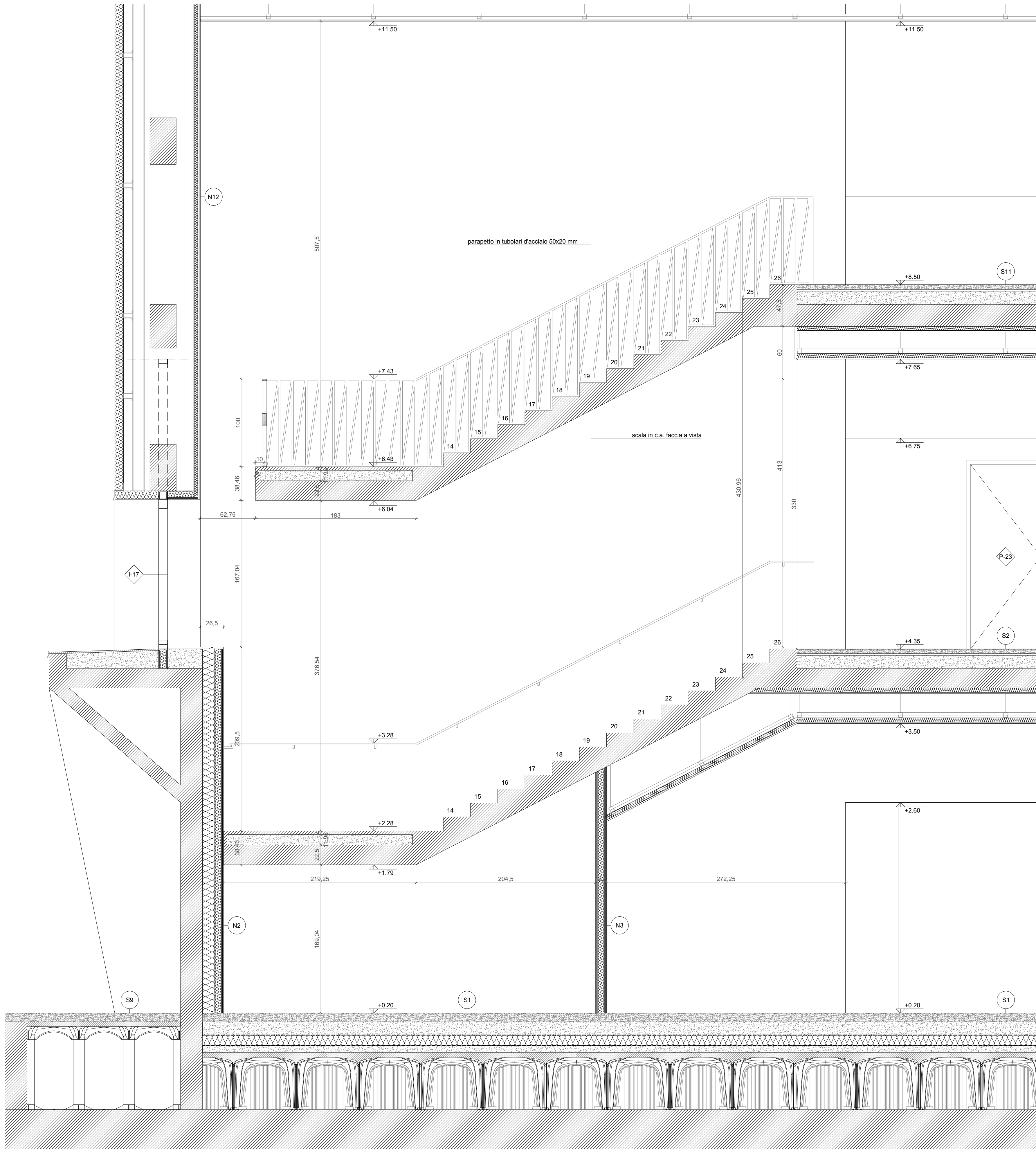
Sezione BB
