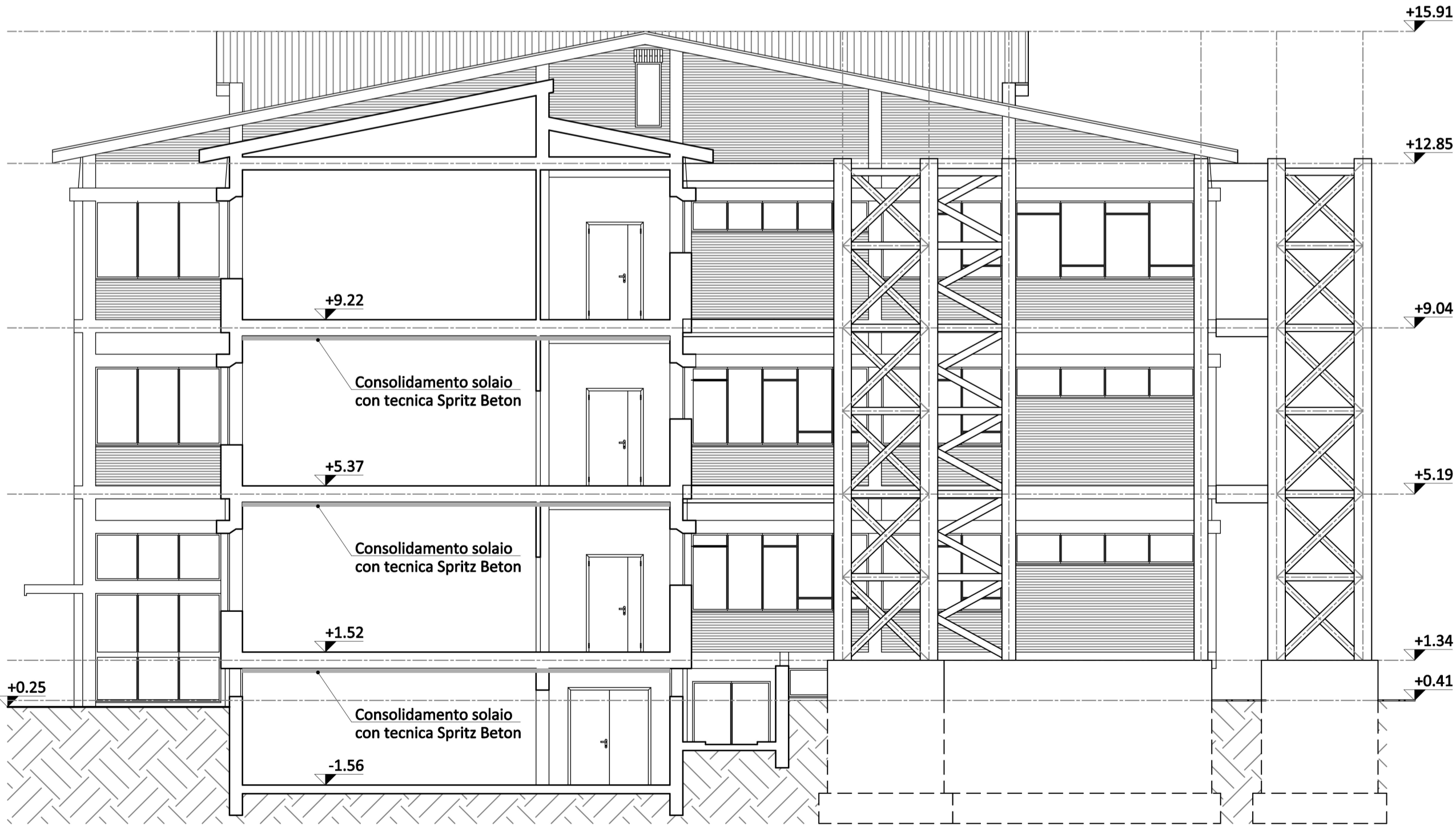
Sezione N-N Scala 1:100
