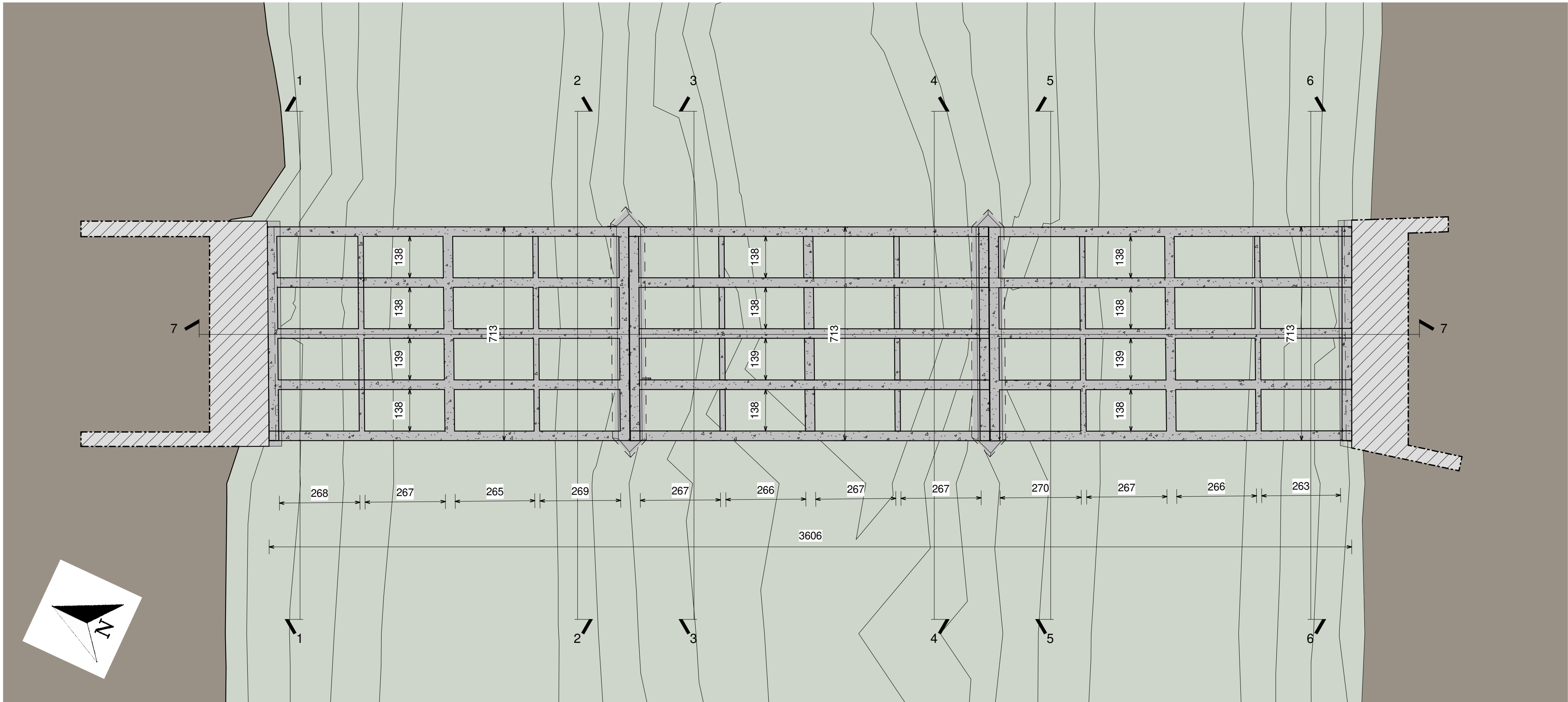
Pianta Travi d'Impalcato
