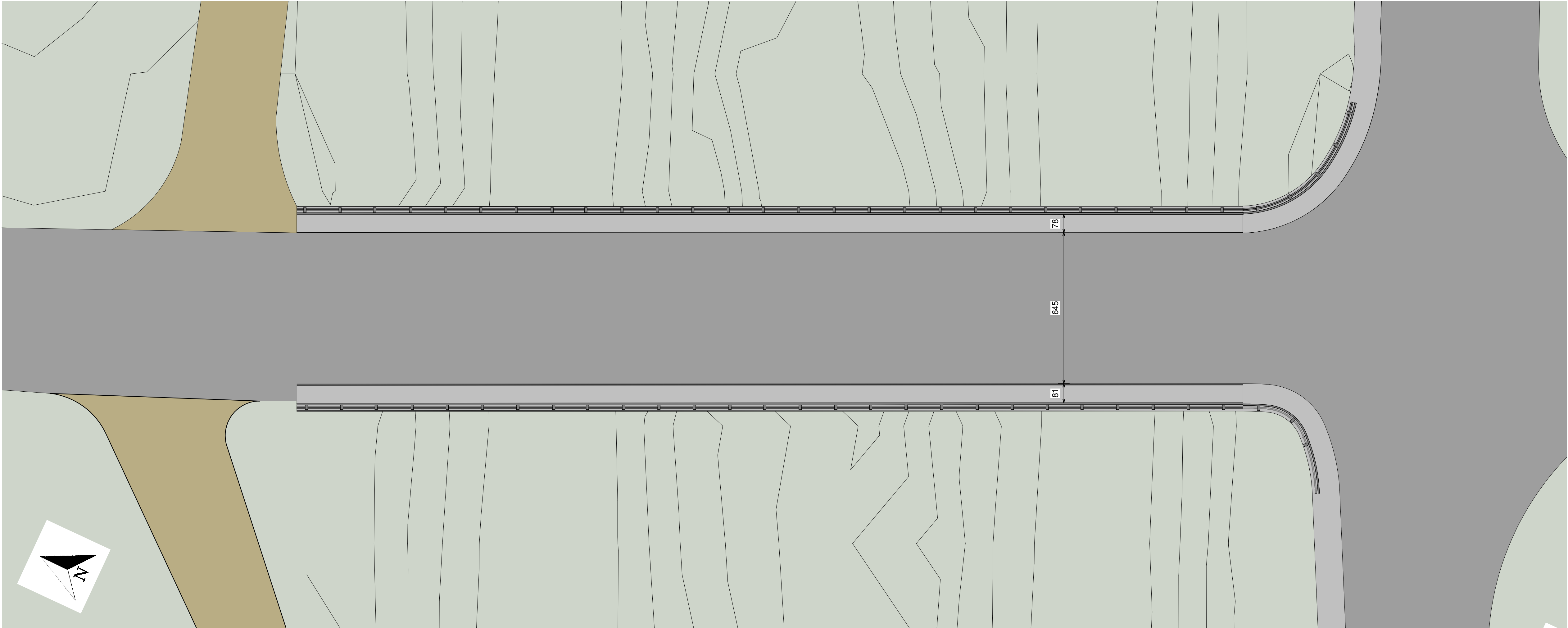
Rilievo - Pianta della sede viaria
