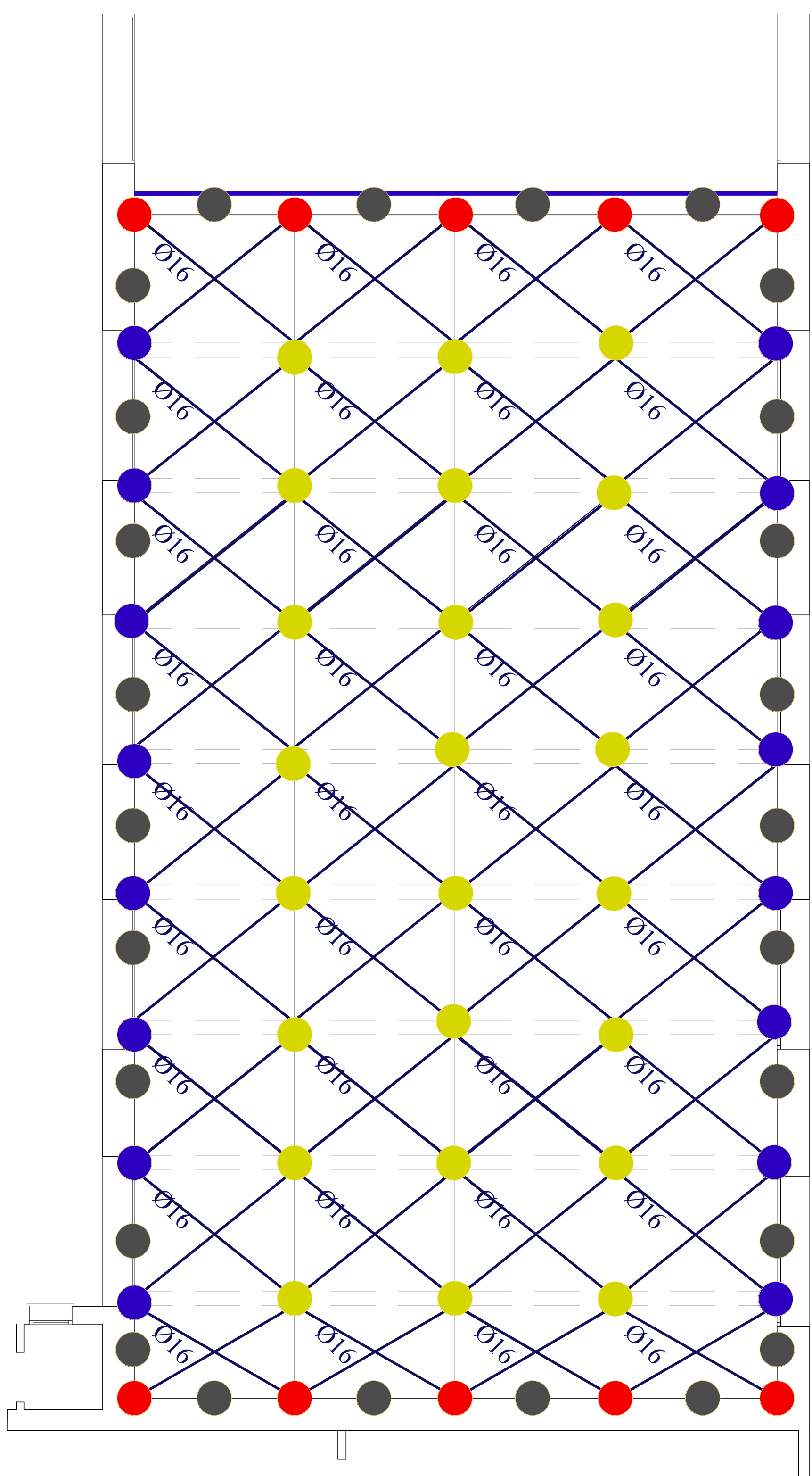
DIAFRAMMA DI PIANO - PIANO SECONDO
