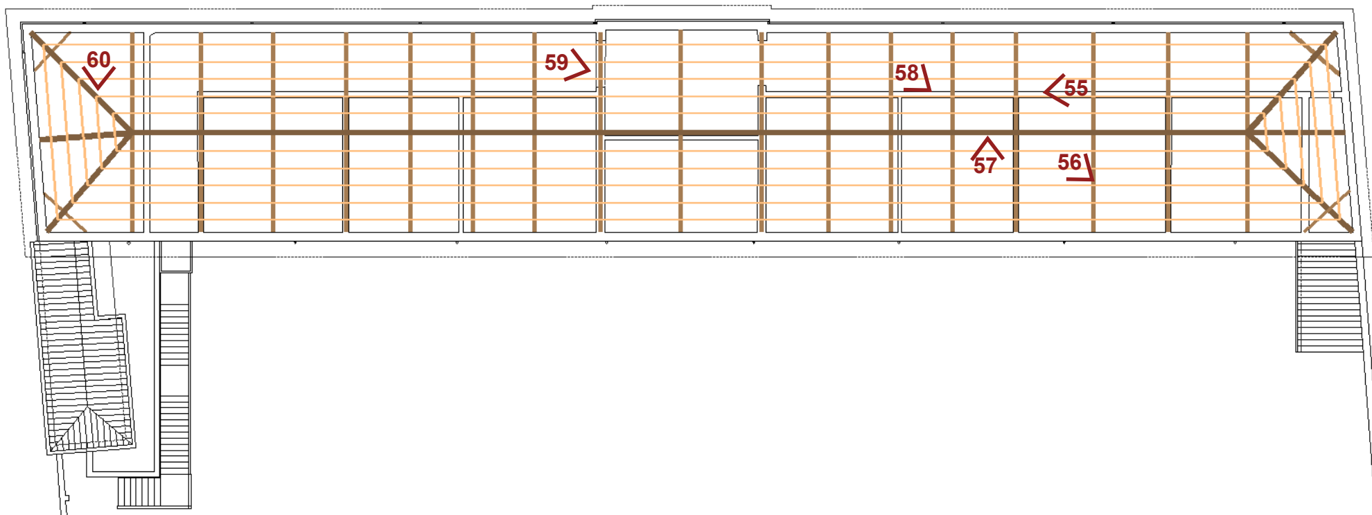
PIANO SOTTOTETTO
