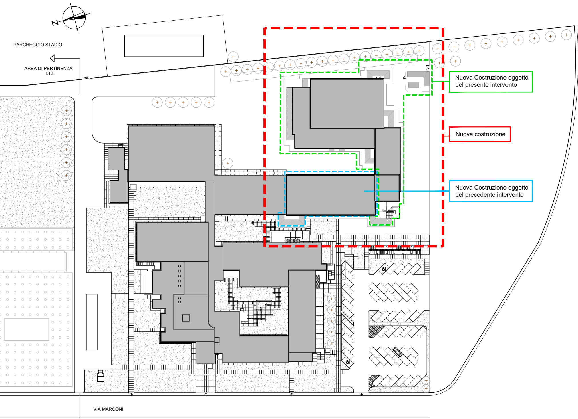
PLANIMETRIA scala 1:1000
