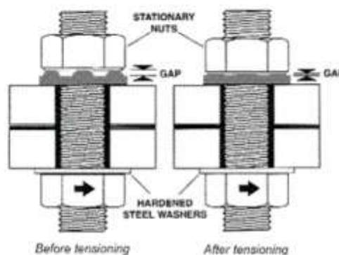
Figura C8.3.2 – Rondelle con indicazione di carico
