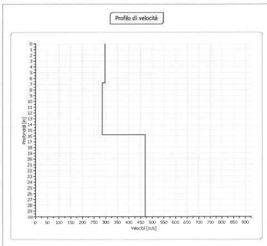
Profilo V_{s30}
